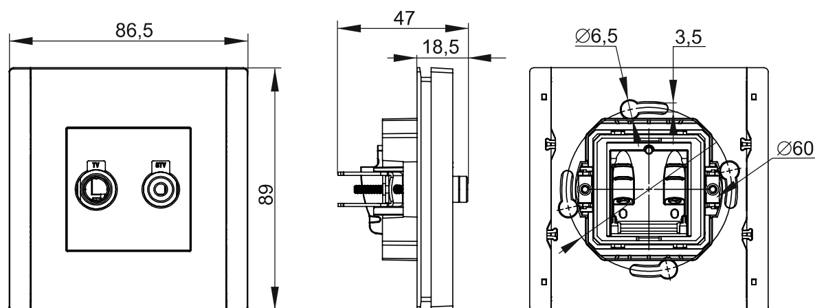
e) TV+SAT розетка / socket / priză / rozetkai
